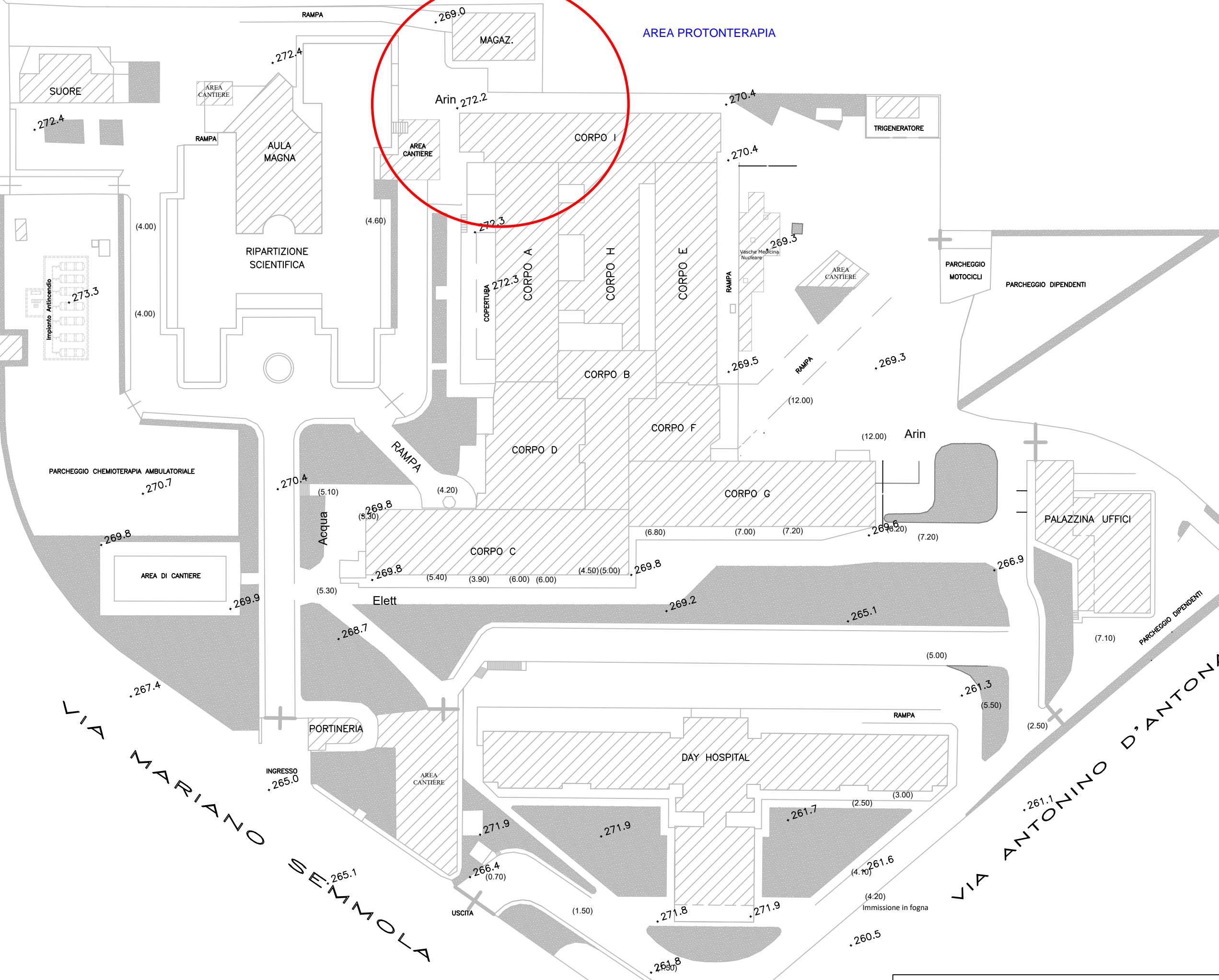
PLANIMTERIA GENERALE DELLE IPOTESI PROGETTUALI
